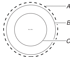
A. Dépassement maximal de 1/2" (1,3 cm) B. Bord extérieur de la table de cuisson C. Taille minimale du plat (le cas échéant)
